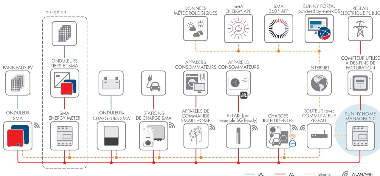
Figure 4 : Topologie avec la solution de stockage SMA et différents appareils consommateurs pilotables (exemple général)
