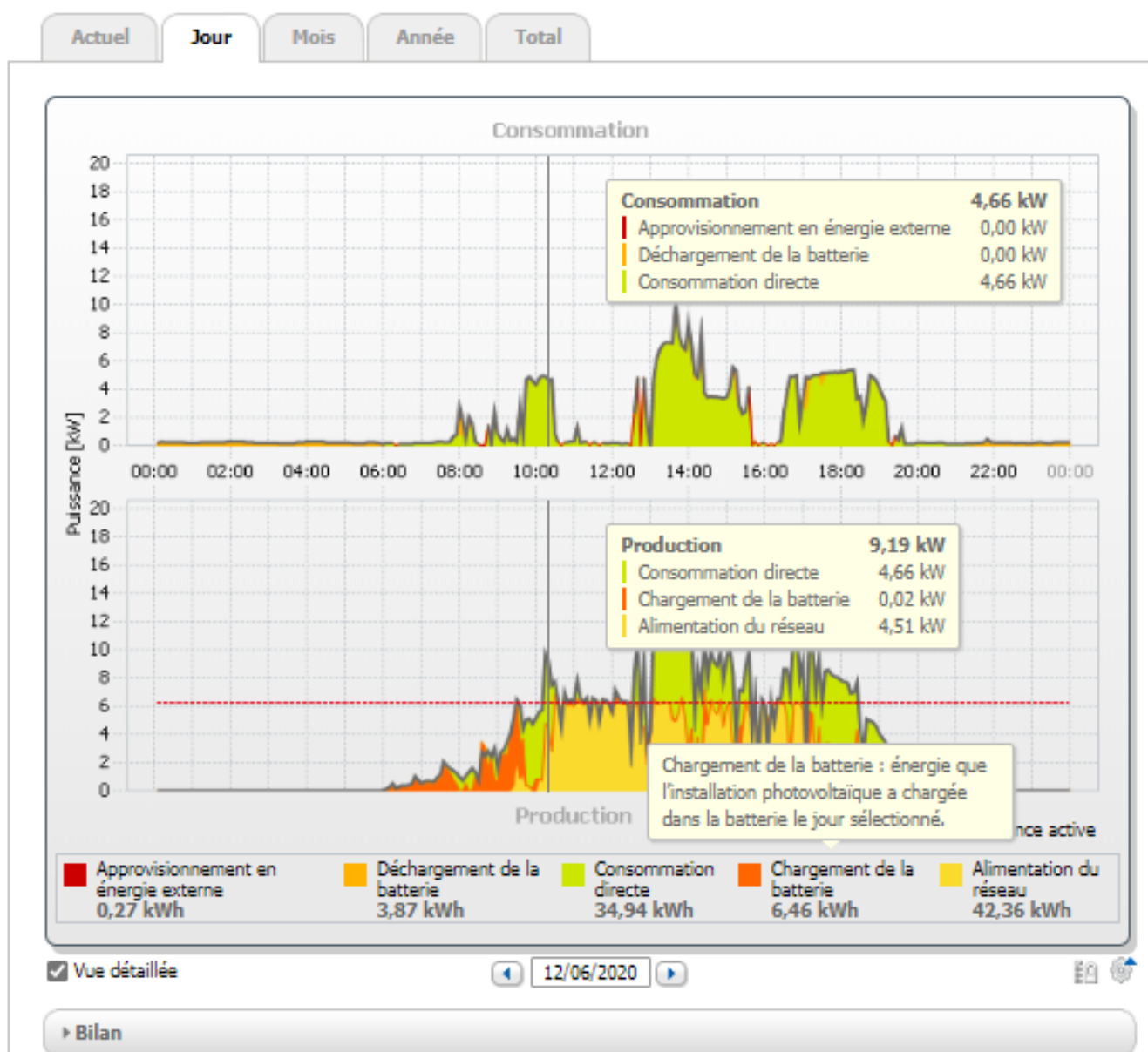
Figure 18 : Bilan énergétique d'un jour déterminé (exemple)
