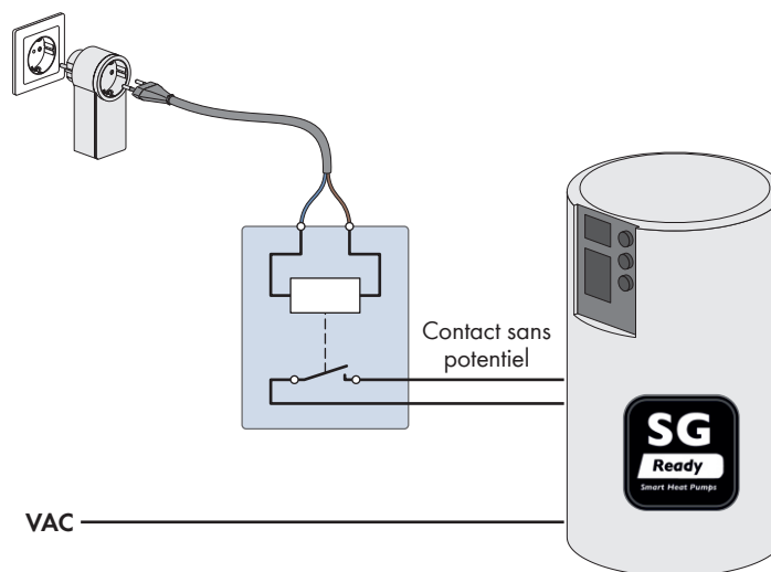
Figure 20 : Raccordement d'une pompe à chaleur via une prise radiocommandée compatible et un relais séparé
